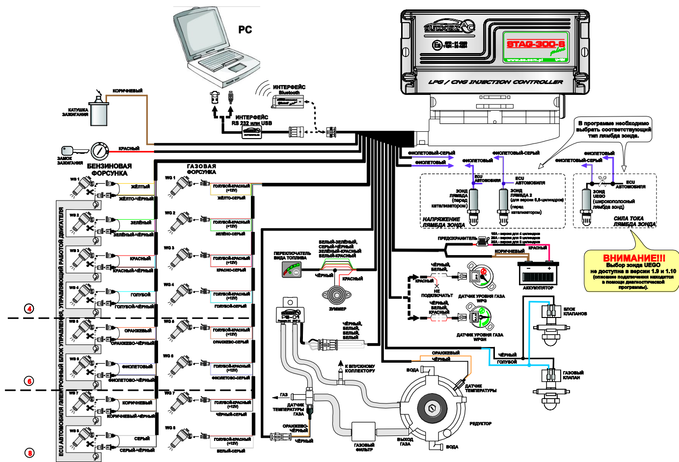
Рис. 3 Схема подключения проводов на автомобиле для STAG-300 Plus.
