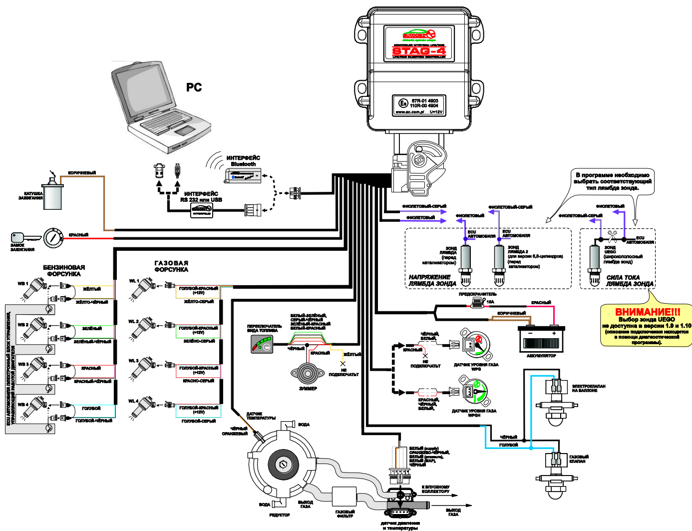
Рис. 2а Схема подключения проводов на автомобиле для STAG-4 (PS-02).
